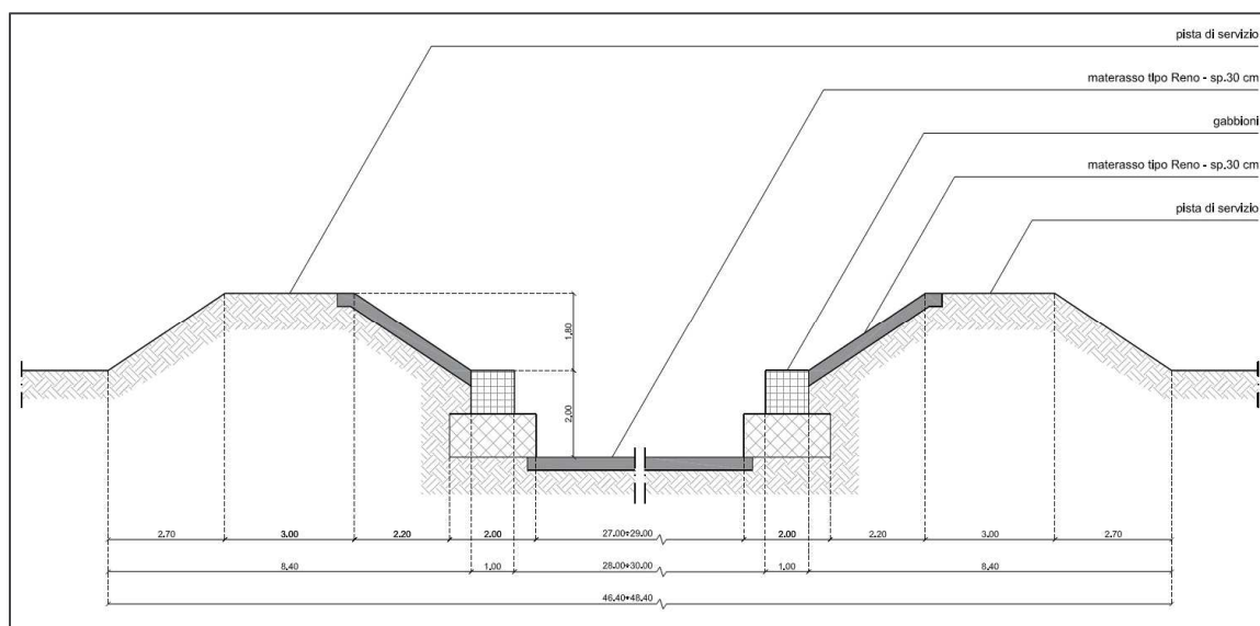
Figura 40 – Sistemazione della nuova sezione idraulica
