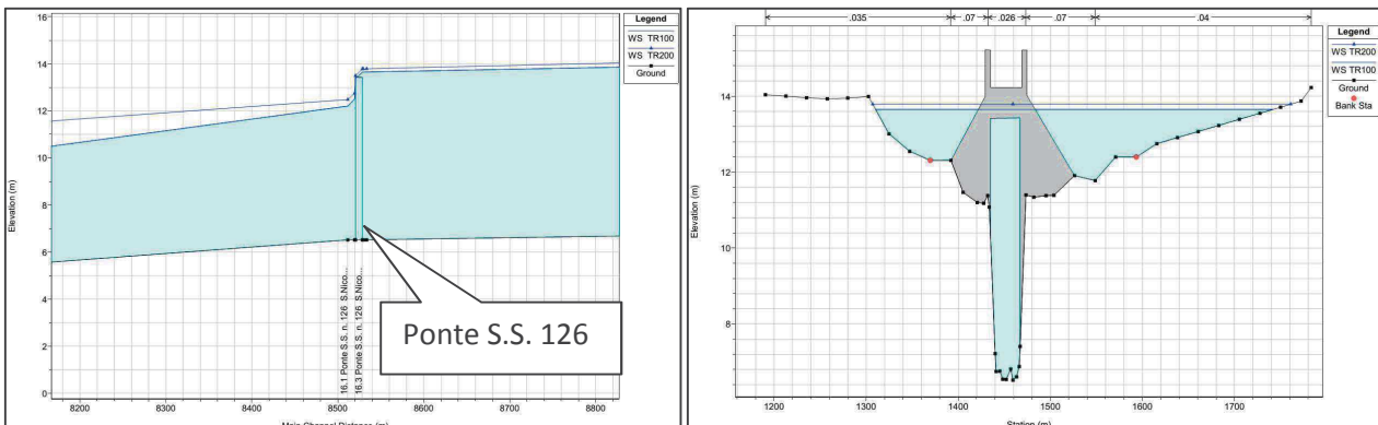
Figura 23 - Profilo longitudinale e sezione idraulica in prossimità del ponte della S.S. 126 – P.S.F.F.
