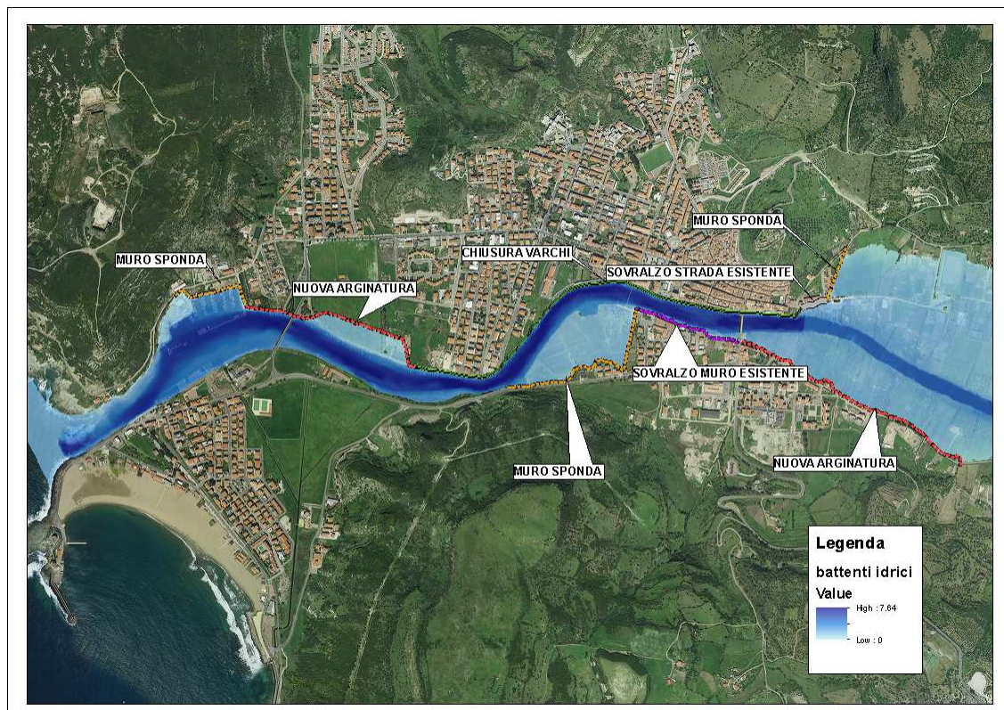
Figura 3.1 – Scenario 2: riduzione dell'estensione allagata (Tr=50 anni)
