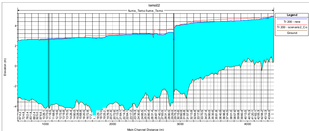
Figura 3.5 - Comparazione tra i livelli idrici relativi alle portate del PSFF (in rosso la condizione exPost).
