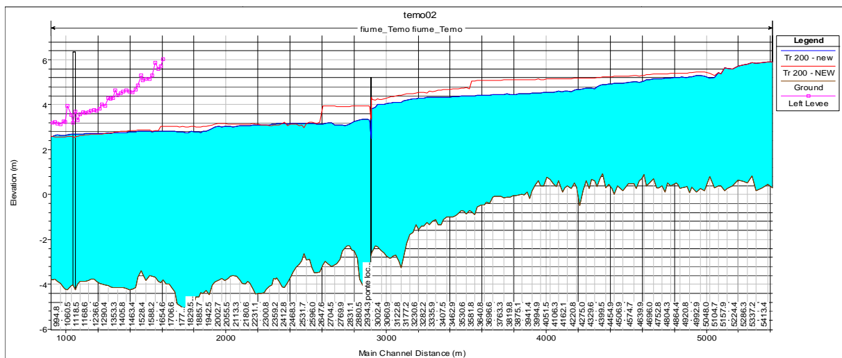
Figura 2.6 - Comparazione tra i livelli idrici relativi alle portate del PSFF (in rosso la condizione exPost).
