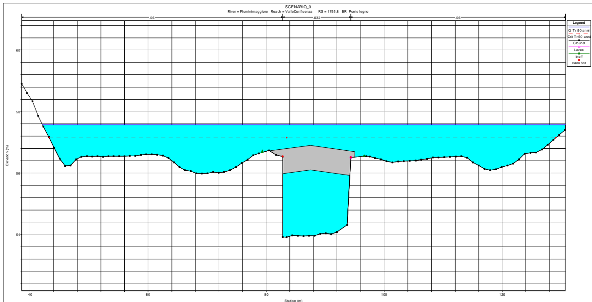
Figura 1.15 – Sezione bagnata in corrispondenza del ponte in legno dell’anfiteatro
