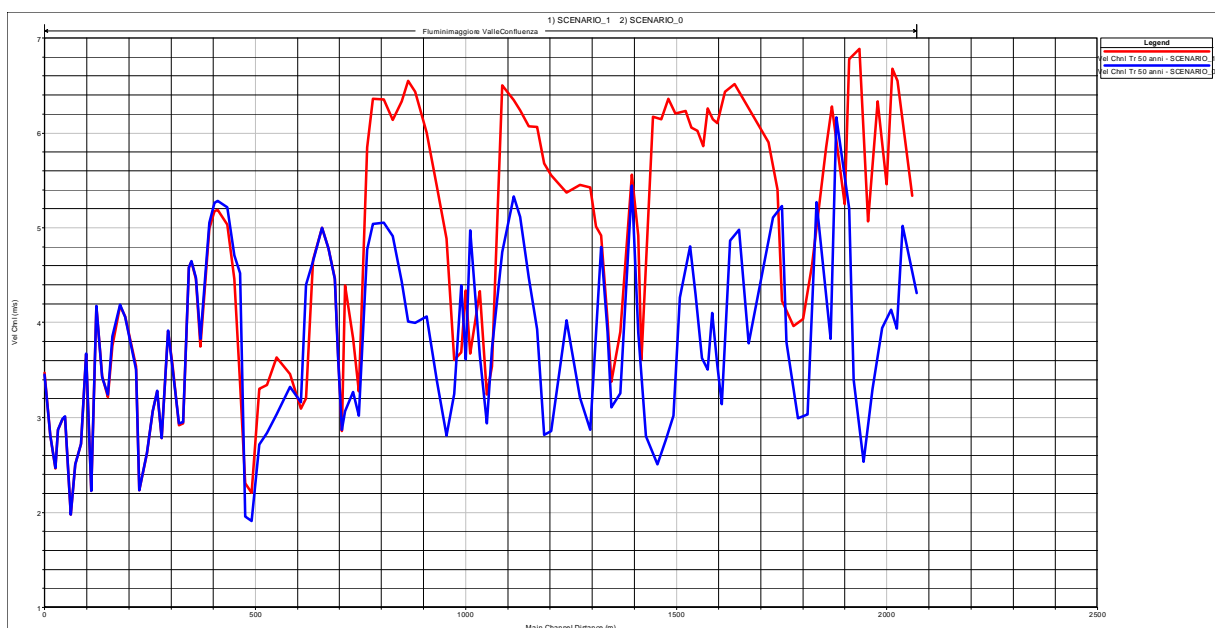
Figura 2.9 – Profilo di velocità lungo il Rio Mannu per lo scenario 1(rosso) e lo scenario 0(blu).
