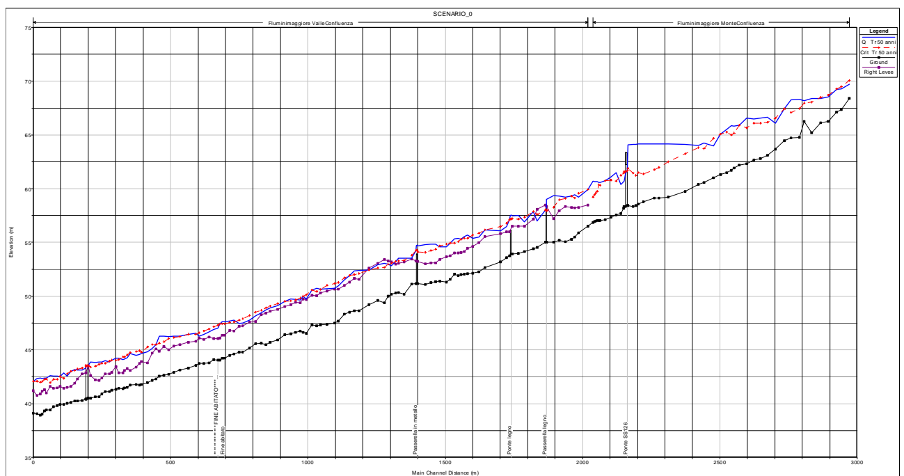
Figura 1.2 – Profilo longitudinale del Rio Mannu allo stato attuale (portata cinquantenaria)
